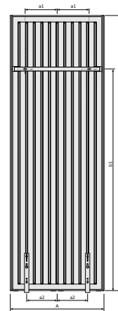
Lodret med MCW6-beslag, set bagfra
